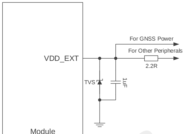
图 38: VDD_EXT 外围参考电路
