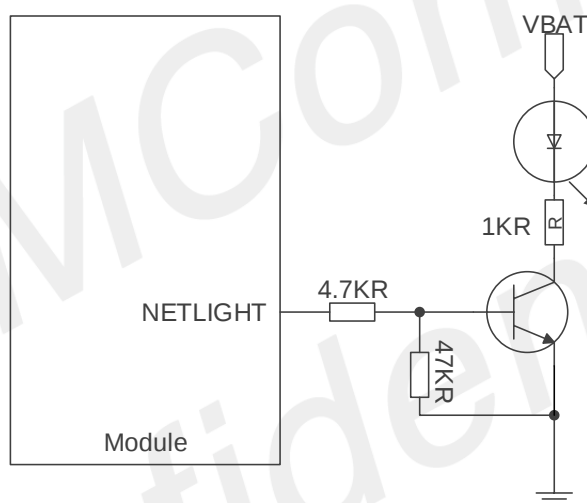
图 31: NETLIGHT 参考电路
