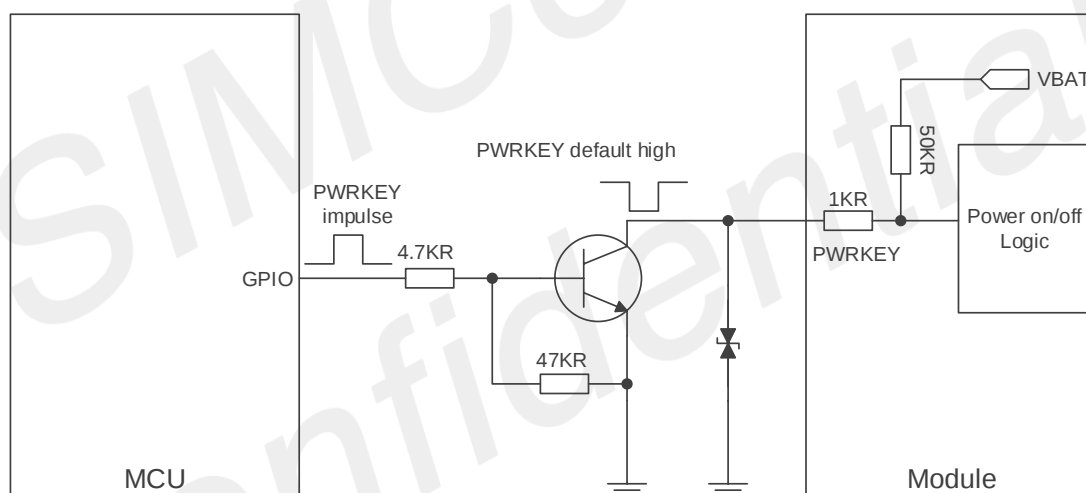
图 9: PWRKEY 参考电路
