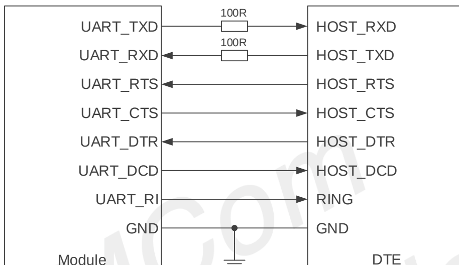
图 14: 串口连接图（全功能模式）
