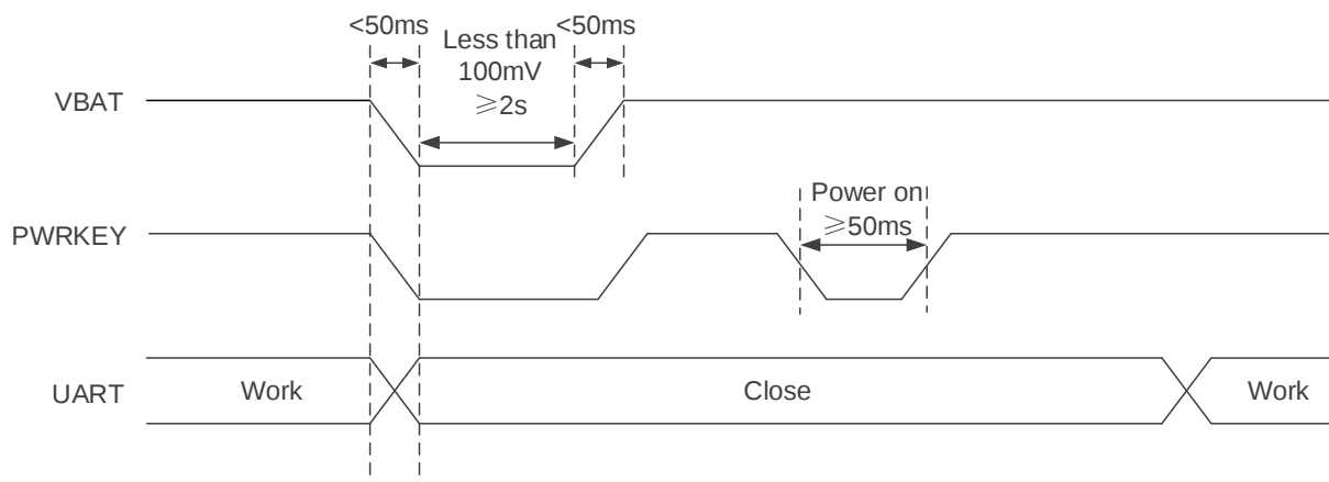
图 8：下电以及上电重启时序
