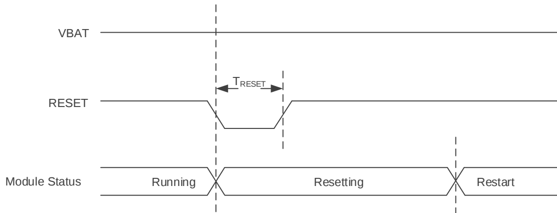
图 13: RESET 复位时序
