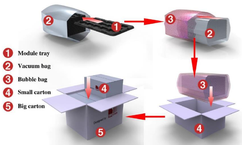
图 48：托盘包装示意图
