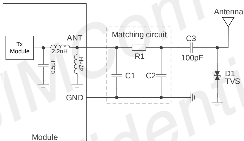
图 39: 无源天线参考电路
