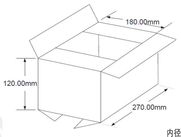
图 50: 小卡通箱尺寸图
