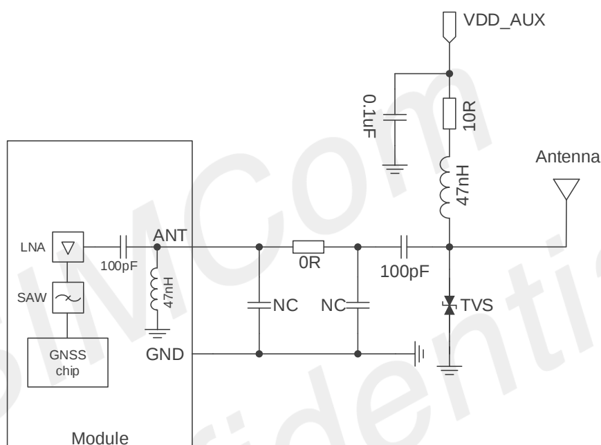
图 40: GNSS 有源天线参考电路
