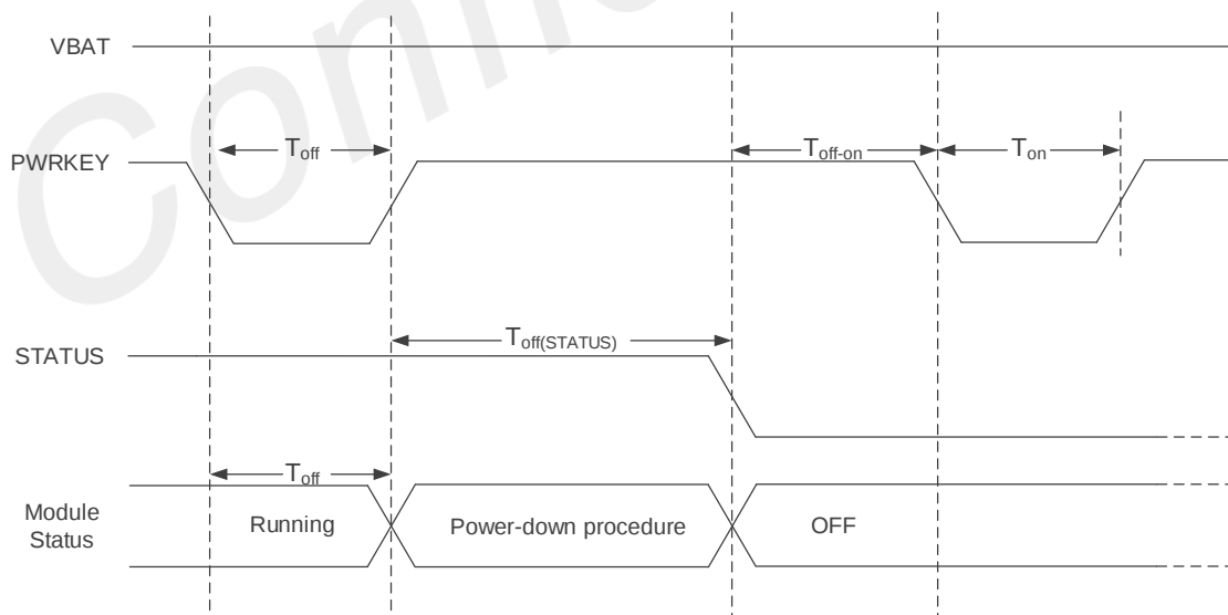
图 11: PWRKEY 关机时序
