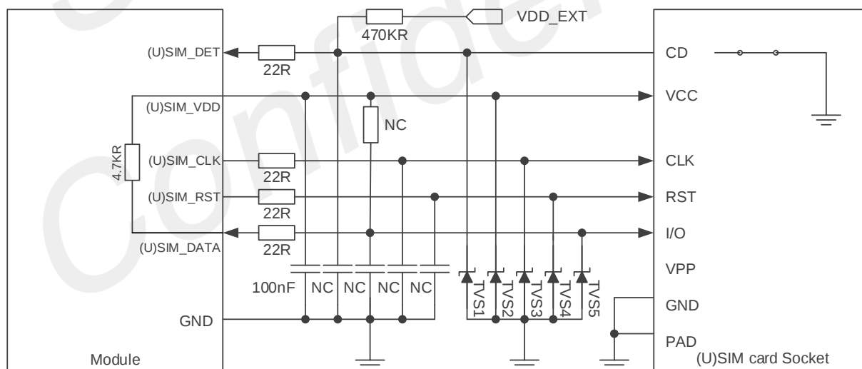
图 22：常闭型 USIM 卡槽参考电路
