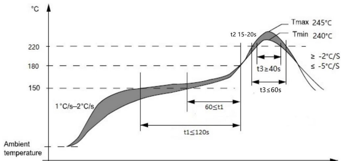
图 46: 推荐的回流焊炉温曲线图（无铅）
