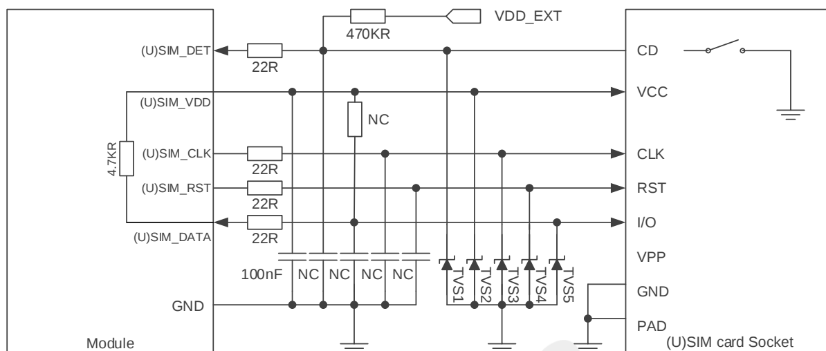
图 23: 常开型 USIM 卡槽参考电路
