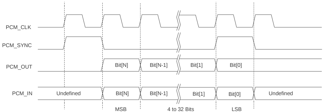
图 24: PCM 短帧同步时序
