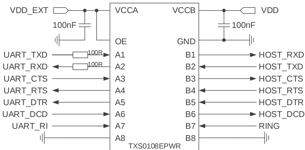
图 16: IC 电平转换参考电路
