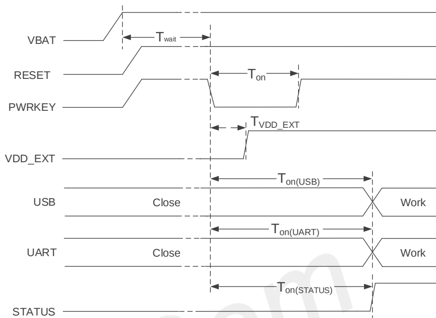
图 10: PWRKEY 开机时序
