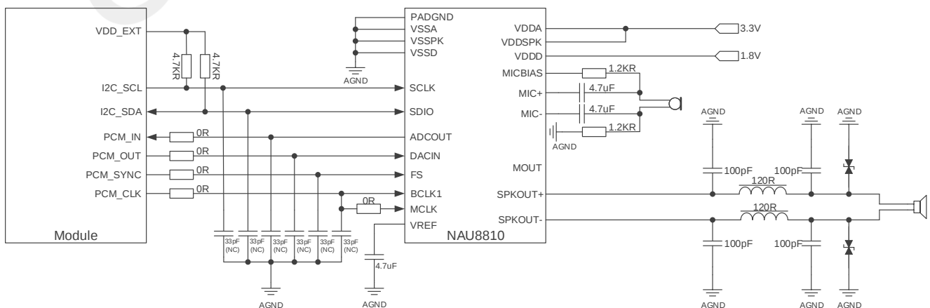
图 26: 数字音频参考电路
