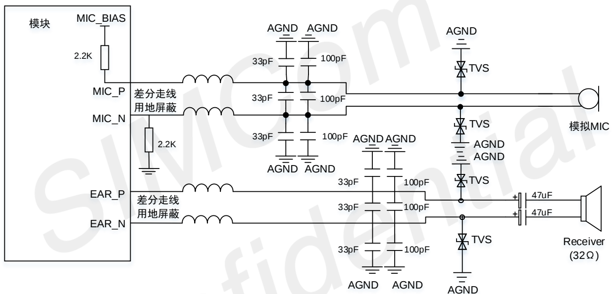
图 27: 模拟音频参考电路
