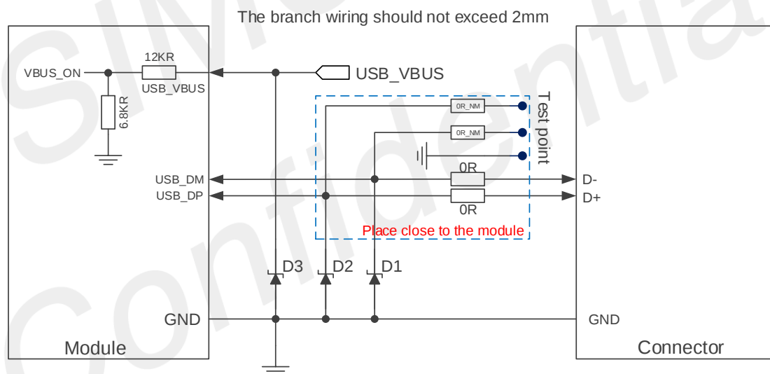
图 19: USB 参考电路
