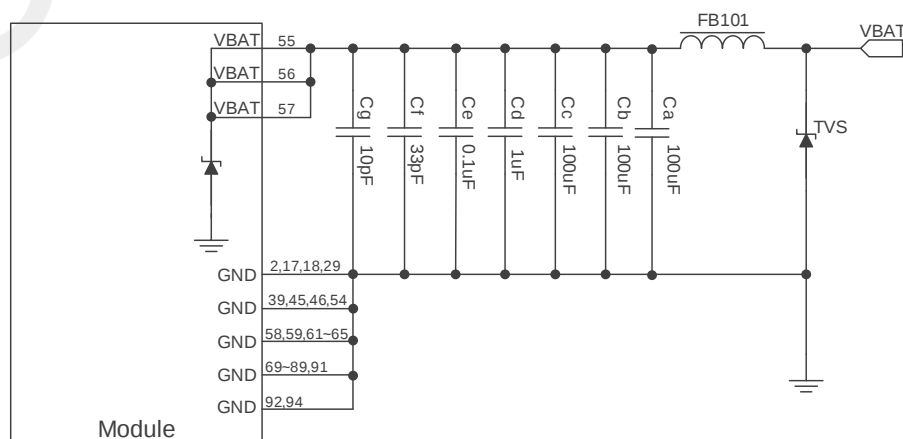
图 6: VBAT 参考电路
