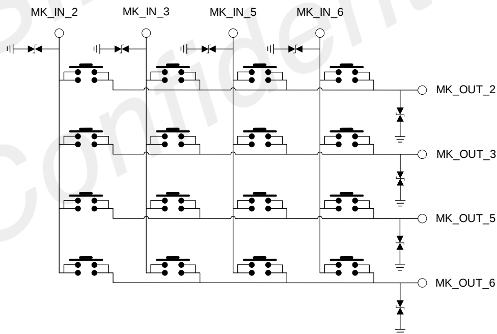
图 28：键盘参考电路
