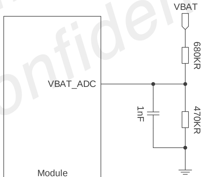
图 37: VBAT_ADC 参考电路
