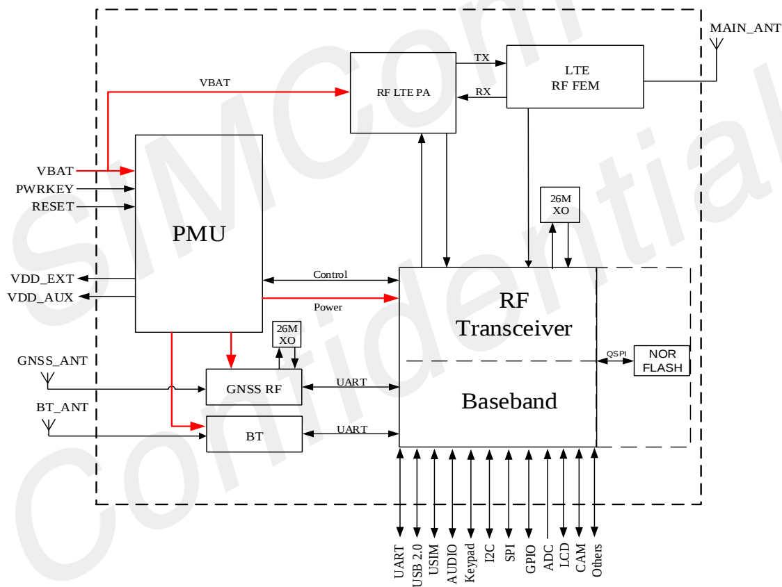
图 1：模块框图
