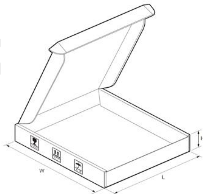
图 54: 卷轴包装箱尺寸图
