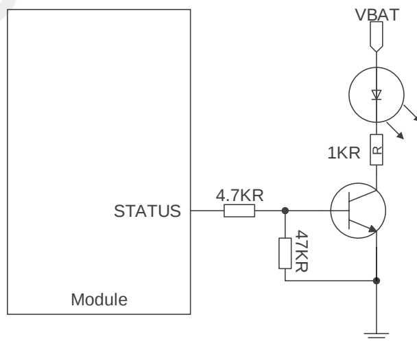
图 32: STATUS 参考电路
