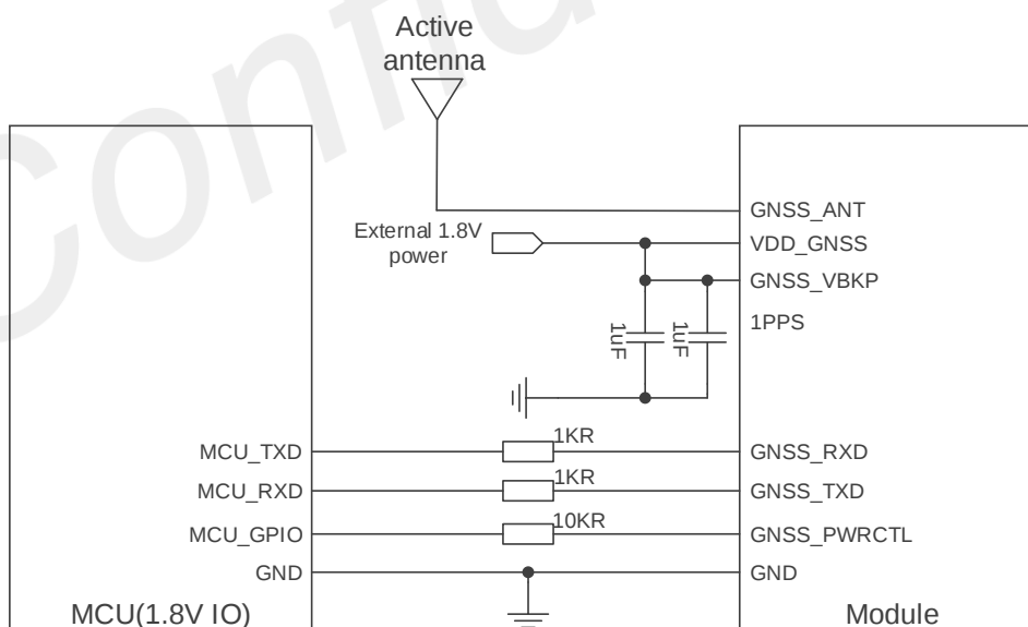
图 34: GNSS 参考电路（独立 GNSS 方案）
