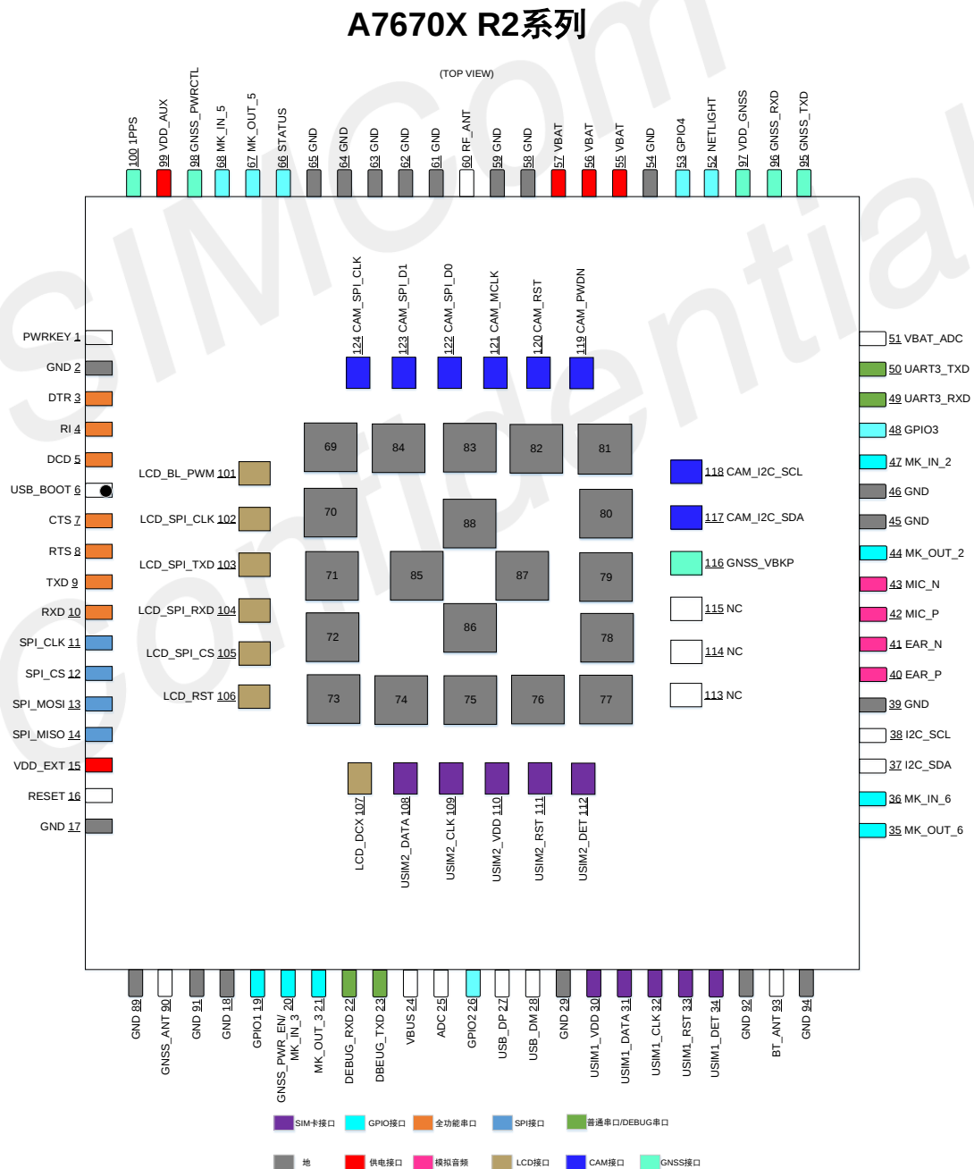
图 2：模块引脚图（正面视图）
