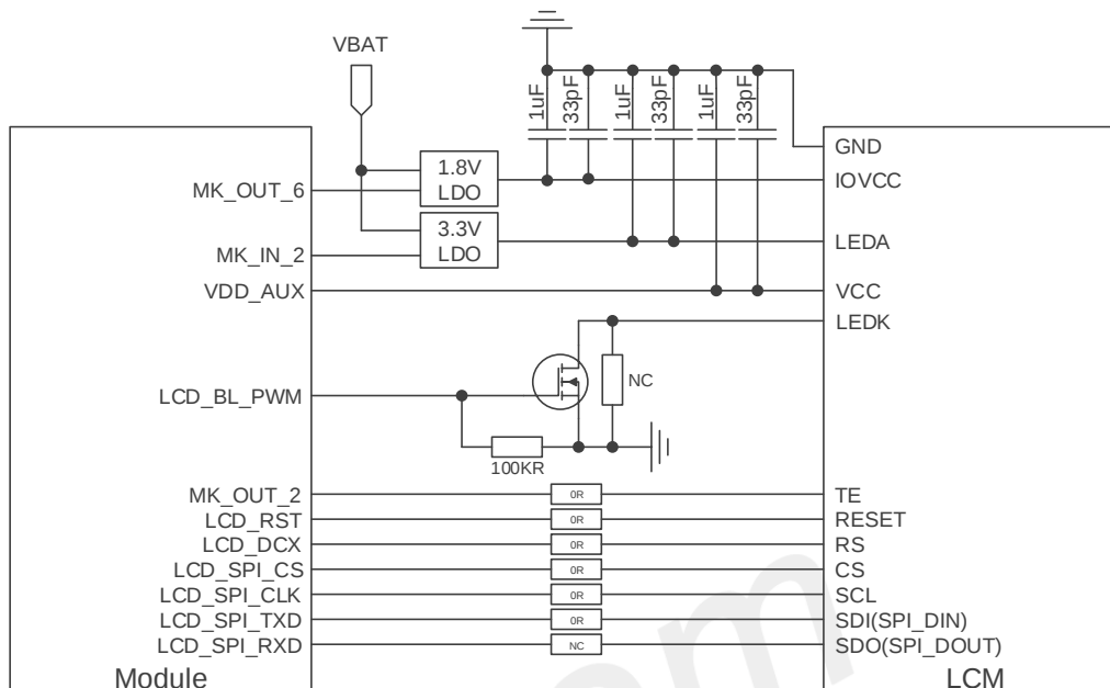
图 35: LCD 参考电路
