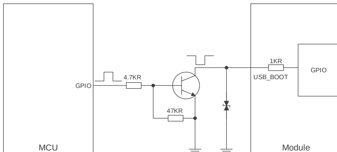
图 20: USB_BOOT 连接图
