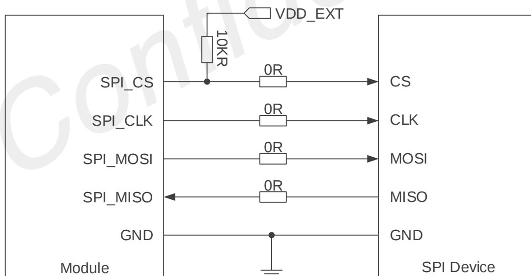
图 30: SPI 参考电路
