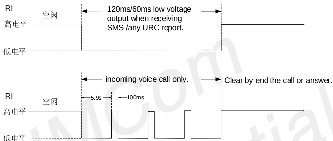
图 18: RI 上电平变化（短信，URC）
