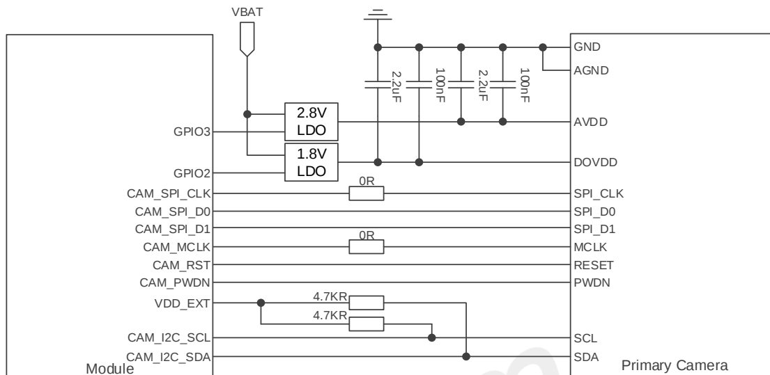
图 36: Camera 参考电路
