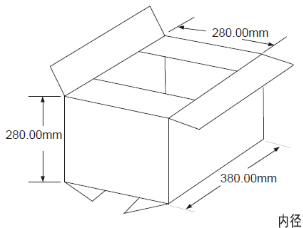
图 51: 大卡通箱尺寸图 (托盘包装)
