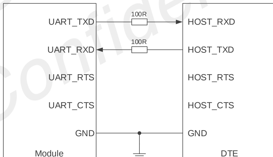
图 15: 串口连接图（NULL 模式）
