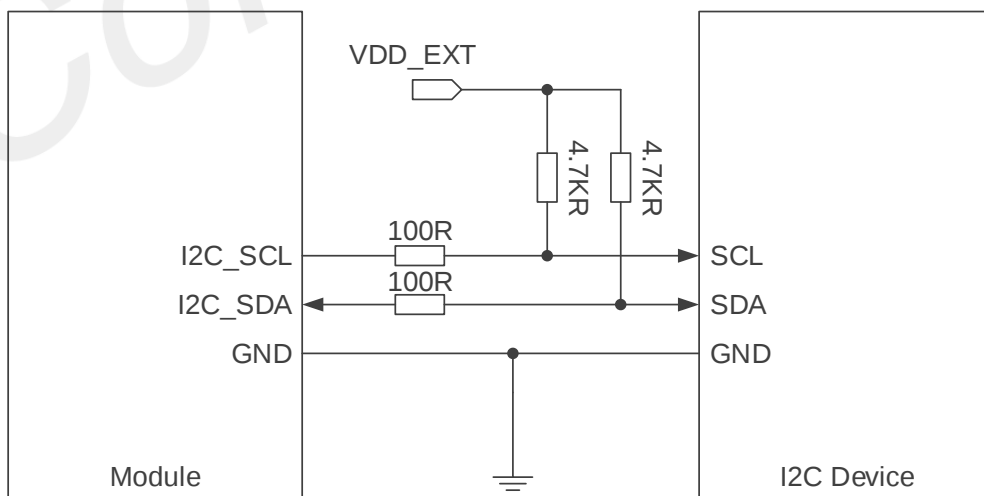
图 29: I2C 参考电路
