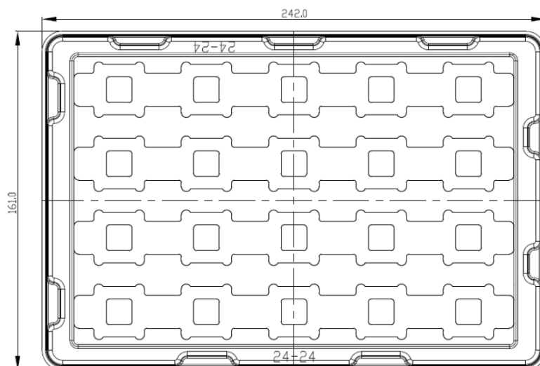
图 49：托盘尺寸图
