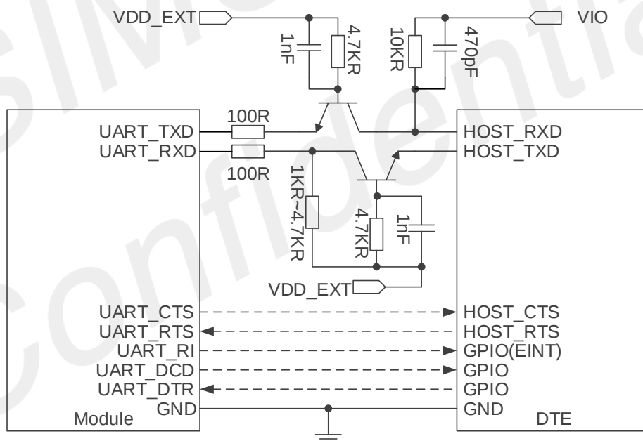
图 17: 三极管电平转换电路
