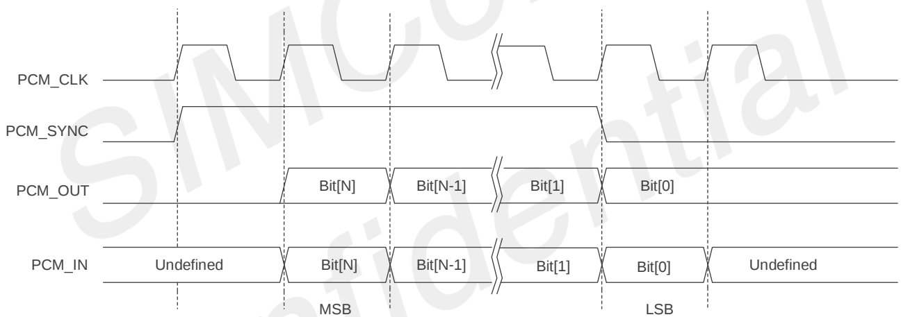
图 25: PCM 长帧同步时序
