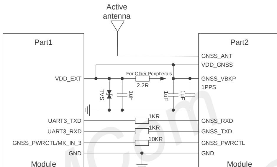
图 33: GNSS 参考电路（非独立 GNSS 方案）
