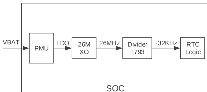
图 43: RTC 框图
