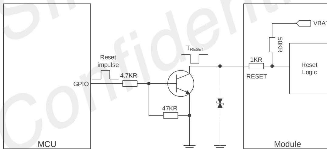
图 12: RESET 参考电路
