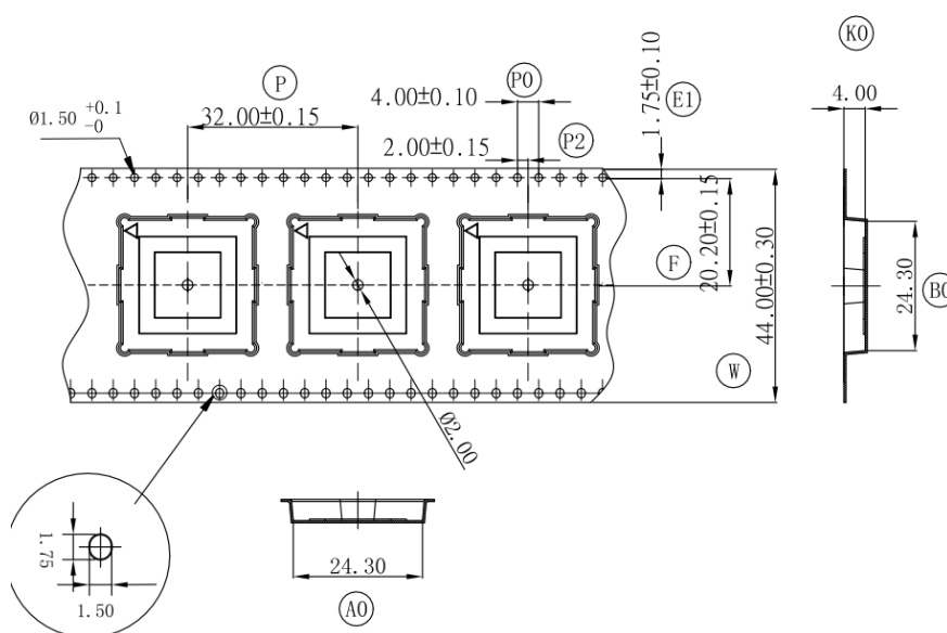
图 53: 卷带尺寸图
